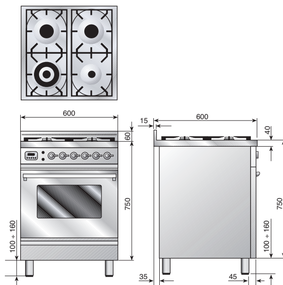
60cm Quadra 4 Burner
